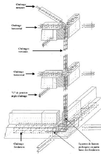
Figures 6.3, 6.4 : Disposition de chaînage parasismique (suivant document Plan Séisme)
