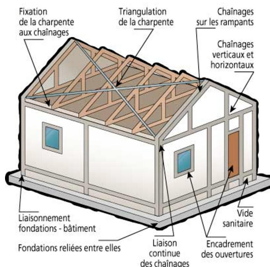
Figures 6.3, 6.4 : Disposition de chaînage parasismique (suivant document Plan Séisme)
