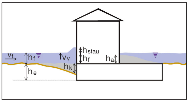
Figure 5.2 : Crues : notations (suivant VKF-AEI)
