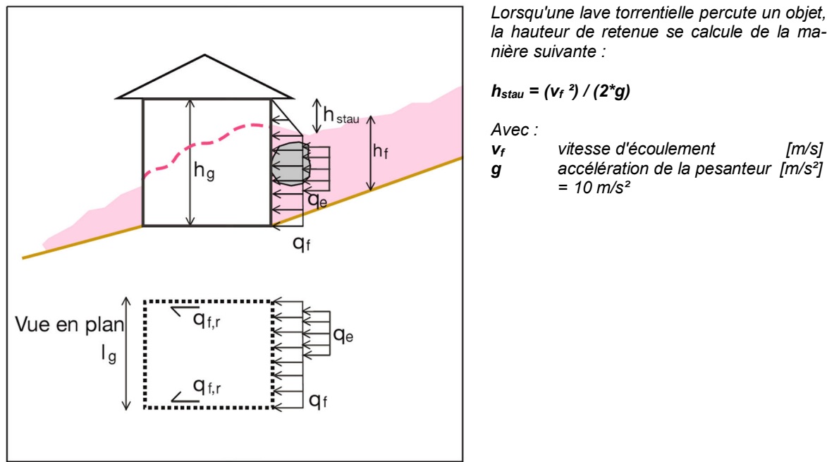
Figure 5.13 : Laves torrentielles : hauteur de retenue due à un obstacle (suivant VKF-AEAI)
