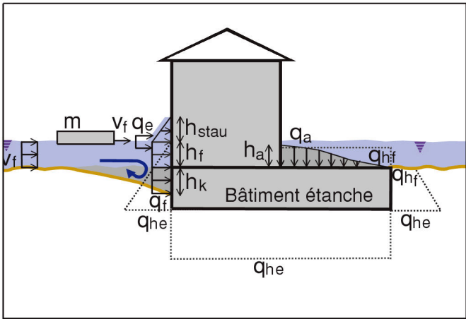
Figure 5.7 : Crues : surcharge due au dépôt de matériaux solides (suivant VKF-AEAI)
