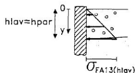
figure 6.13 : diagramme des poussées par unité de surface
