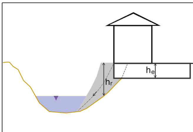
Figure 5.10 : Crues : glissement de la berge (suivant VKF-AEAI)
