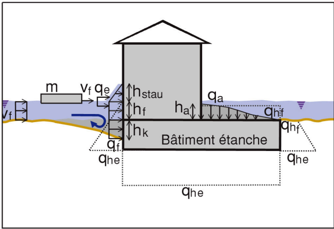
Figure 5.8 : Crues : force de choc due à des charges concentrées (suivant VKF-AEAI)
