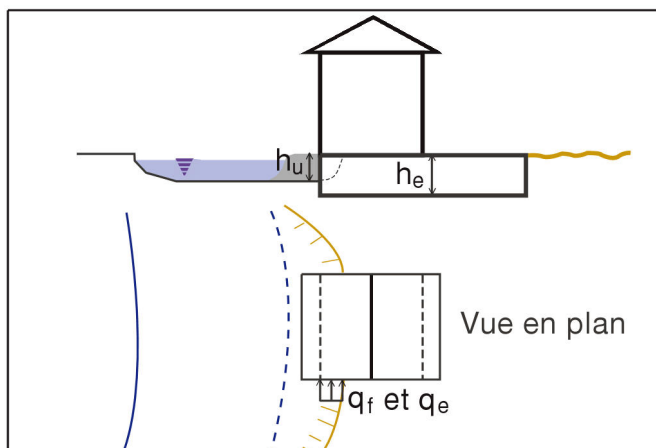
Figure 5.9 : Crues : déplacement du lit du cours d'eau (suivant VKF-AEAI)
