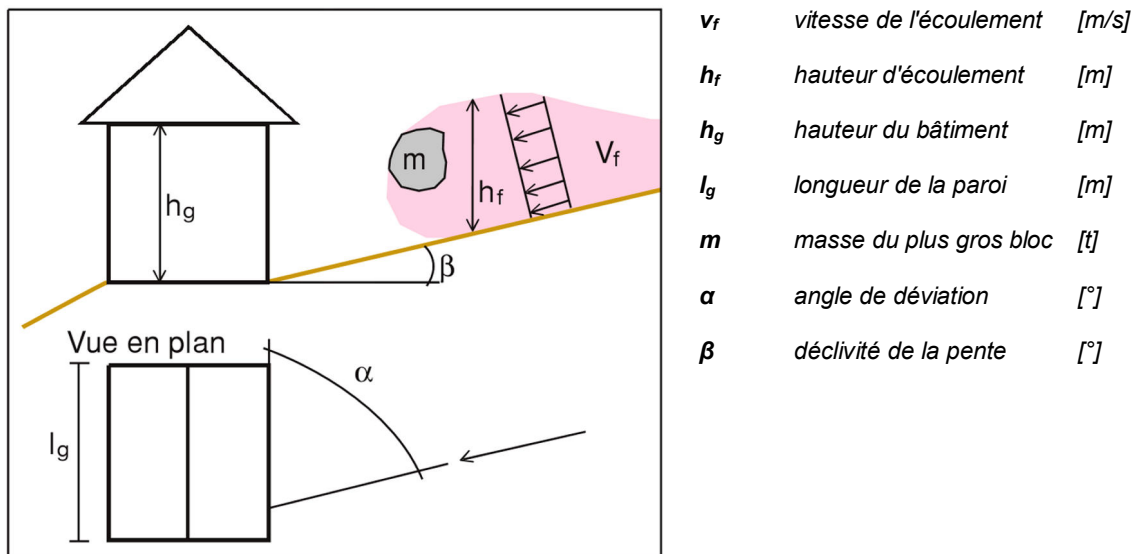
Figure 5.11 : Laves torrentielles : notations (suivant VKF-AEI)
