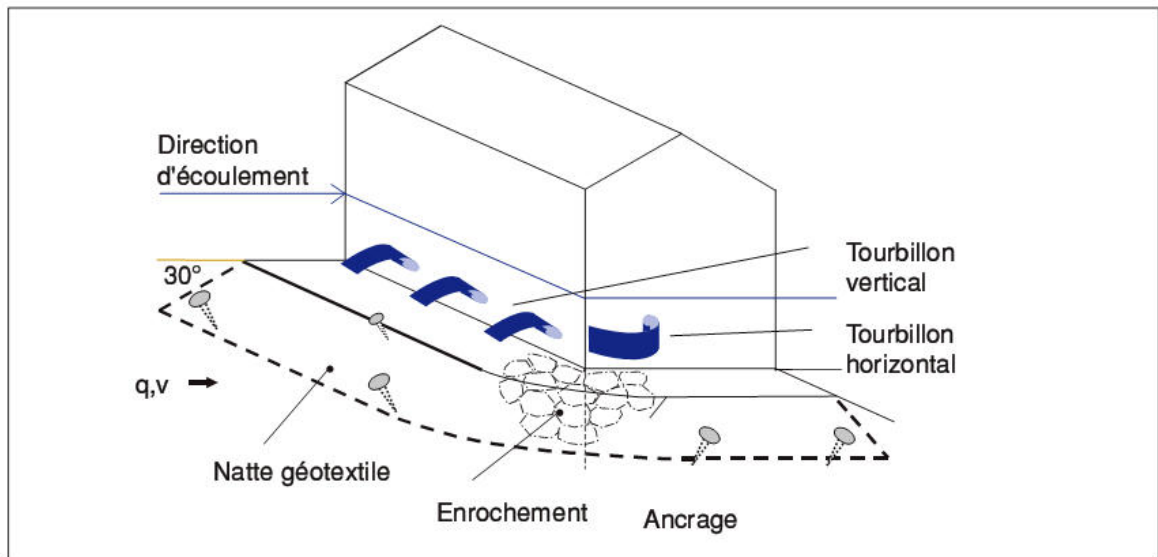
Figure 6.2 : Protection des fondations contre l'affouillement (suivant assurances suisses VKF-AEAI)
