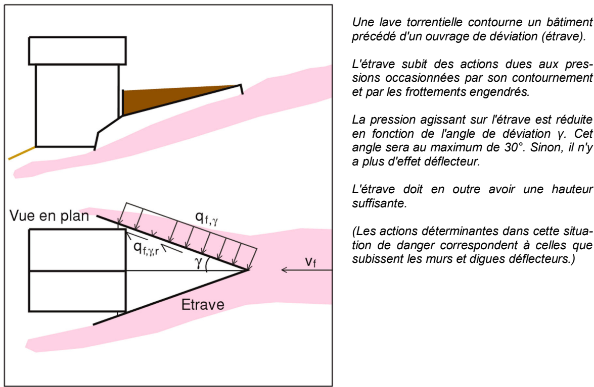
Figure 5.16 : Laves torrentielles : bâtiment précédé d'un ouvrage de déviation (suivant VKF-AEAI)
