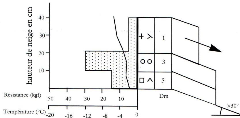
Figure 4.3 Type de représentation en usage en Suisse (IFENA) et aux États-Unis. La flèche indique qu'il y a eu un décrochement de la couche superficielle. La déclivité est indiquée également.
