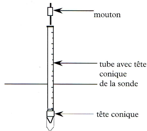
Figure 4.1 Schéma de principe d'une sonde de battage
