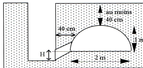
Figure 9.13 Igloo creusé dans la neige. C'est la tranchée qui sert de fosse à froid.
