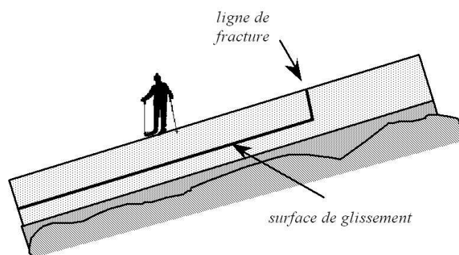
Figure 5.25 La plaque est mise en mouvement après la rupture par traction le long de la ligne de fracture et par cisaillement sur la surface de glissement. La rupture initiale (primaire) peut être selon les mécanismes l'un ou l'autre de ces processus.
