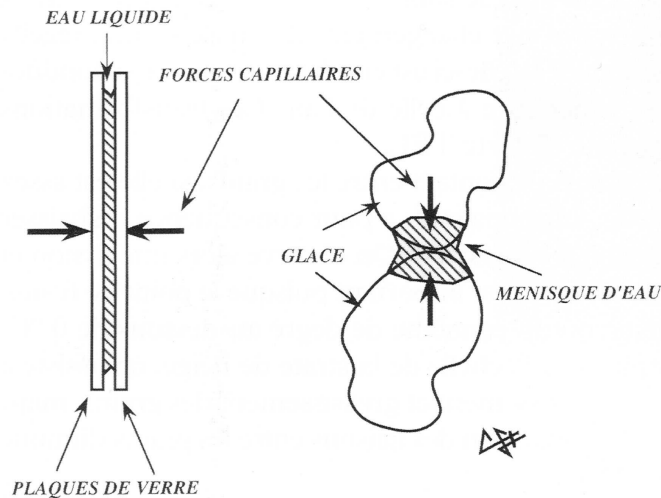
Figure 3.10 Lorsque l'on accole deux plaques de verre mouillées, on constate qu'il est très difficile de les séparer ensuite. Les forces capillaires se développent au sein du filin d'eau liquide et s'exercent sur les plaques. C'est le même phénomène qui se produit lorsque deux grains de neige humides sont en contact. L'eau liquide forme un ménisque autour du point de contact et les forces capillaires tendent à les maintenir accolés.
