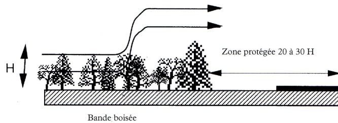
Figure 8.7 Effets d'une bande boisée. D'après [8].
