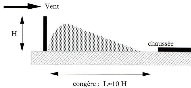
Figure 8.4 Effet dû à une barrière imperméable. D'après [8].
