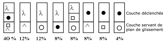
Figure 5.27 Les différents types de neige dans la couche déclenchée et la nature de la couche de glissement lors d'accidents concernant des skieurs (avalanches non spontanées). La configuration de loin la plus dangereuse semble être une couche de neige en cours de métamorphose (particules reconnaissables puis grains fins) sur une couche de gobelets ou de faces planes. Analyse réalisée sur un échantillon de 25 avalanches accidentelles [26].
