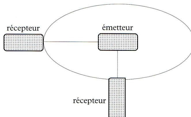
Figure 9.19 La portée est la plus grande quand les appareils émetteur et récepteur sont parallèles à leur axe longitudinal et devient la plus faible lorsqu'ils sont placés selon un axe perpendiculaire.
