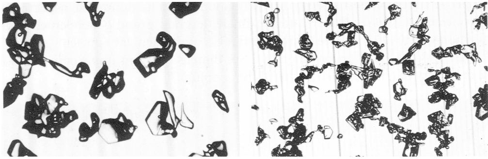
Figure 3.7 Grains à faces planes photographiés à différents grossissements. Les traits verticaux sont espacés de 0,2 mm. Photographies Météo-France/CEN/Edmond PAHAUT.
