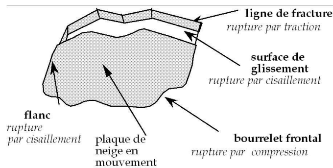
Figure 5.24 Terminologie des ruptures. Les frontières de la plaque de neige sont définies par la rupture de la couche déclenchée, qui se fait en une succession d'étapes dont l'ordre dépend du mécanisme.
