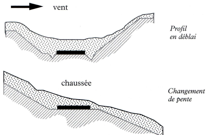
Figure 8.8 Profils propices au développement des congères. D'après [8].
