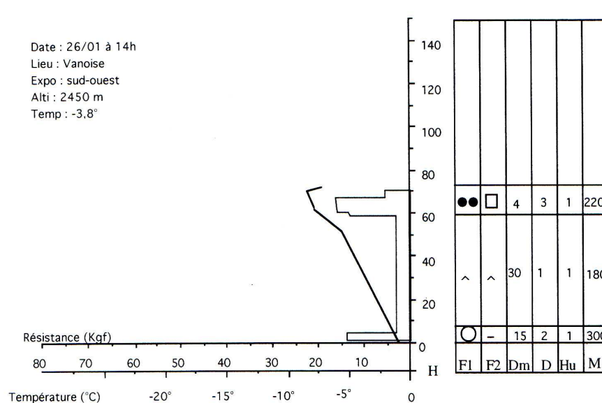
Figure 4.4 Profil réalisé dans le massif de la Vanoise par beau temps le 26 janvier à 14h à 2450 m. Le profil met en évidence l'existence d'une plaque de faible épaisseur (10 cm), composée de grains fins (neige légèrement ventée?) et de grains à faces planes (métamorphose de gradient moyen due aux conditions anticycloniques régnant depuis plusieurs jours). Cette plaque repose sur une épaisse couche de gobelets (50 cm) de faible cohésion. Cette couche d'épaisseur importante date probablement de décembre (temps sec et froid). Le gradient de température est encore important (jusqu'à 0,18^\circ /cm entre 40 et 50 cm). On peut considérer ce manteau comme instable compte tenu de la superposition d'une plaque dure (solidité moyenne, faible épaisseur) sur une grosse couche de faible cohésion: il a provoqué la mort d'un skieur retrouvé enseveli sous 1,50 m de neige. D'après [3].
