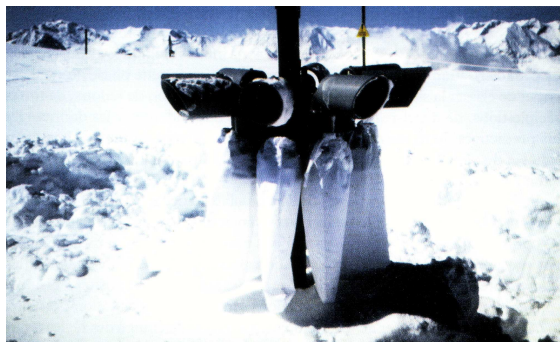
Figure 7.7 Le driftomètre, appareil renseignant sur le transport de neige par le vent (direction et intensité). Ce matériel a été mis au point en soufflerie puis testé en situation réelle. Il fournit une donnée hautement prédictive des avalanches dues au transport éolien.
