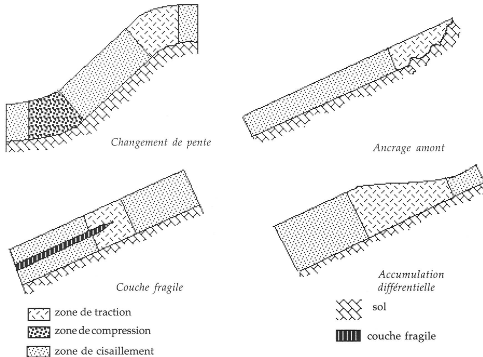
Figure 3.14 Schémas de principe de l'apparition des zones où le cisaillement devient important et conditionne l'instabilité éventuelle du manteau.
