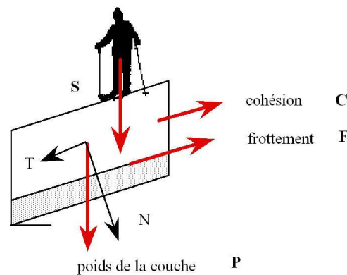
Figure 5.23 Lors du passage d'un skieur, le frottement F et la cohésion C doivent compenser l'augmentation de la composante tangentielle du poids pour que l'équilibre persiste.
