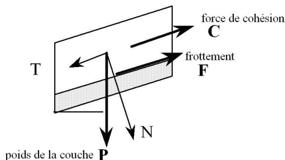
Figure 5.22 La strate supérieure est soumise à trois forces : le poids P , les forces de cohésion et le frottement F . Elle est en équilibre si le frottement F et la cohésion C contrebalancent la composante tangentielle T du poids.
