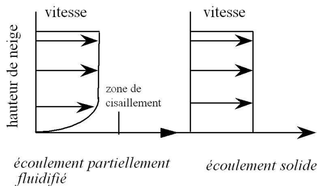
Figure 5.35 Les deux familles d'écoulements denses classés selon leur profil de vitesse.
