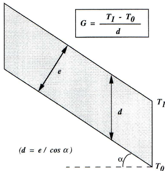
Figure 3.4 Méthode du calcul du gradient vertical de température pour une couche de neige située sur une pente.
