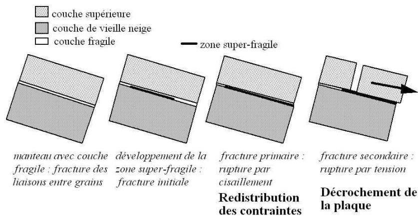
Figure 5.29 Les différentes étapes d'une rupture amenant à un départ en plaque : la rupture de la surface de frottement au niveau de la couche fragile provoque une redistribution soudaine des contraintes.
