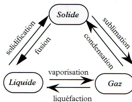
Figure 2.2 Désignation des différents types de changements de phase selon le sens de ce changement.
