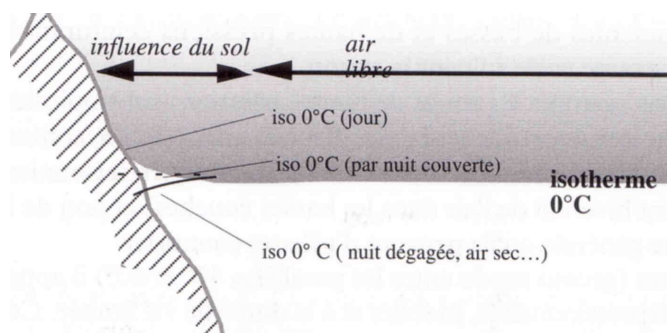
Figure 2.3 Température au sol et isotherme 0°C en fonction des conditions météorologiques et de l'heure.
