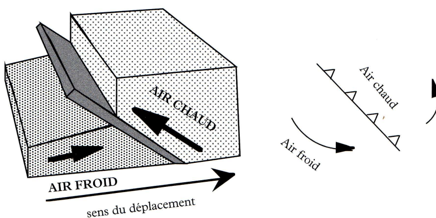
Figure 2.8 Dans le cas du front froid, l'air chaud est chassé par l'air froid et rejeté violemment en altitude. La surface frontale est fortement inclinée, le front s'étend sur quelques dizaines de kilomètres. Le principe de représentation est identique au cas précédent. Le front froid est schématisé comme indiqué sur la figure. D'après [1].
