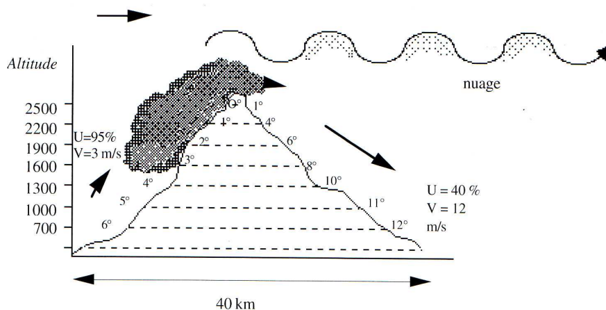
Figure 2.12 Effet de foehn. De l'air chaud et humide remonte une pente. En se refroidissant, la vapeur d'eau se condense et forme des nuages, qui peuvent donner des précipitations. L'air libéré de son humidité provoque un vent chaud et sec sur l'autre versant. C'est l'effet de foehn. Le passage de la crête provoque un sillage, qui donne naissance à des nuages lenticulaires. À titre indicatif, on donne la variation de température de chacun des versants, ainsi que la perte d'humidité (relative U ) du vent dont la vitesse moyenne croît.
