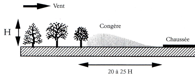
Figure 8.6 Rôle d'une haie brise-vent. D'après [8].
