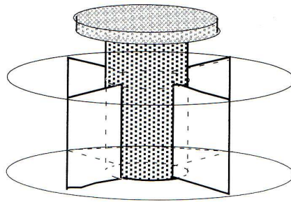
Figure 6.3 Scissomètre. La rotation des pales de l'arbre crée une surface de cisaillement de forme cylindrique. On mesure le couple de frottement exercé par l'échantillon à la rupture pour déduire la résistance au cisaillement.
