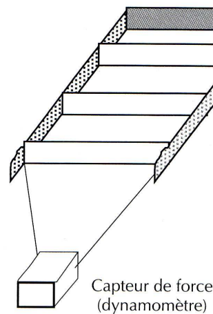
Figure 6.4 Le cadre de cisaillement est composé d'un cadre rigide maintenant des peignes. On tire, tout en mesurant la force nécessaire à l'aide d'un dynamomètre, sur le cadre placé long de la couche dont on souhaite étudier les propriétés. On peut mesurer la force de rupture pour différentes charges normales ; pour cela il suffit de placer différentes charges de neige dans les espaces entre les peignes. La surface de cisaillement est généralement comprise entre 100 et 500 cm 2 .
