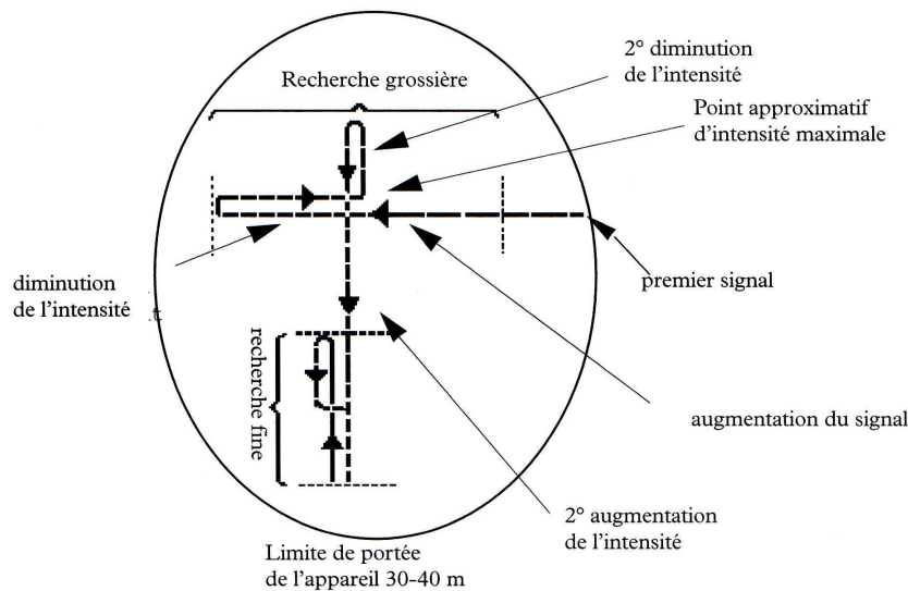
Figure 9.17 Recherche par angles droits.
