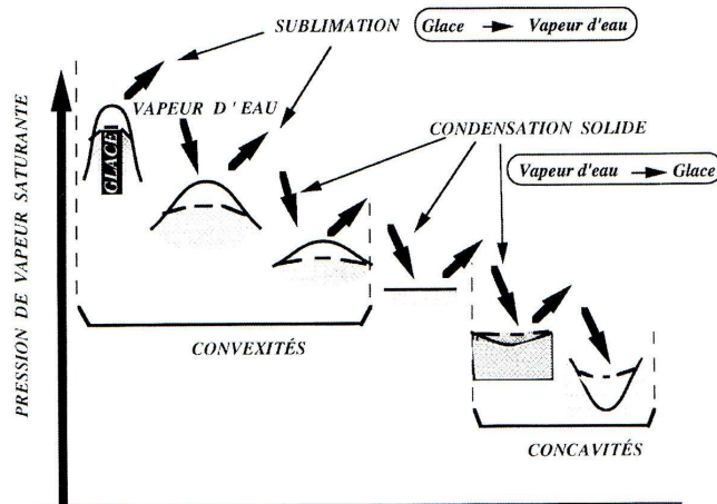
Figure 3.2 Schéma des transferts de glace, par la phase vapeur, des surfaces les plus convexes vers les surfaces moins convexes et concaves.
