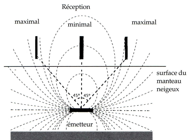
Figure 9.18 Cas où l'ARVA se situe au milieu des deux extrema. Un cas analogue se produit lorsque l'appareil est placé verticalement.
