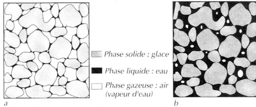
Figure 3.12 Schéma de la répartition des trois phases de l'eau, dans le cas des faibles TEL (a) et dans le cas des fortes TEL (b).
