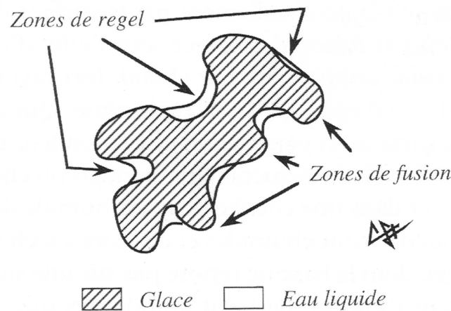
Figure 3.11 Schéma montrant, pour un grain de neige, les zones de fusion (convexités et les zones de regel (concavités)).
