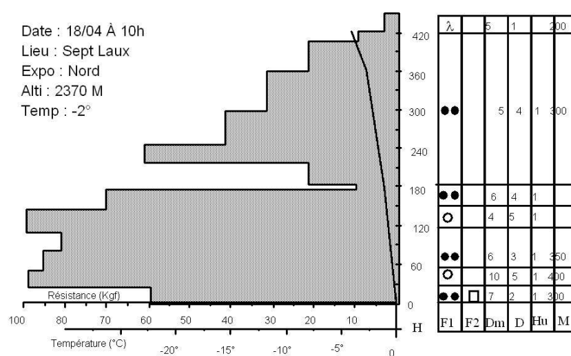
Figure 5.20 Histogramme de résistance au battage et profil stratigraphique d’après un sondage du CEN réalisé le lendemain à l’endroit du décrochement.
