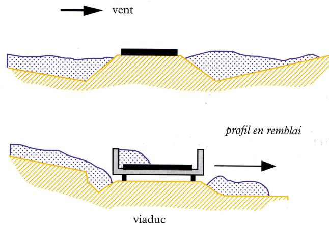
Figure 8.9 Aménagements en vue de réduire les congères. D'après [8].
