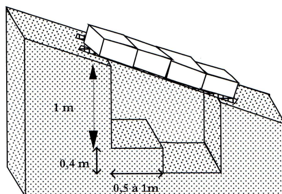
Figure 9.11 Schéma de réalisation du trou dans la neige (banquette et fosse à froid).
