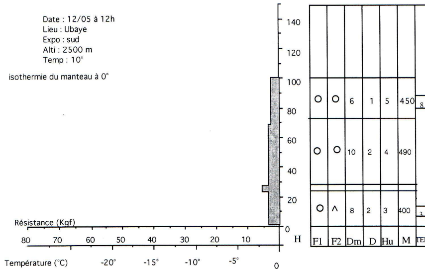
Figure 4.5 Profil réalisé dans la vallée de l’Ubaye par beau temps le 12 mai à 12h à 2500m d’altitude. L’ensemble du manteau est de faible cohésion et largement humidifié. La TEL est supérieure à 6 % sur la quasi-totalité du manteau, ce qui indique le « pourrissement » de l’ensemble du manteau qui est déjà ancien (la masse volumique approche dans la partie médiane les 500 \text{ kg/m}^3 ). Le risque d’avalanche (mobilisant de la neige lourde) n’est pas négligeable. D’après [3].
