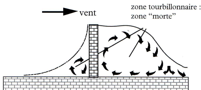
Figure 2.15 Effet d'un obstacle sur un écoulement d'air : création de zones mortes.
