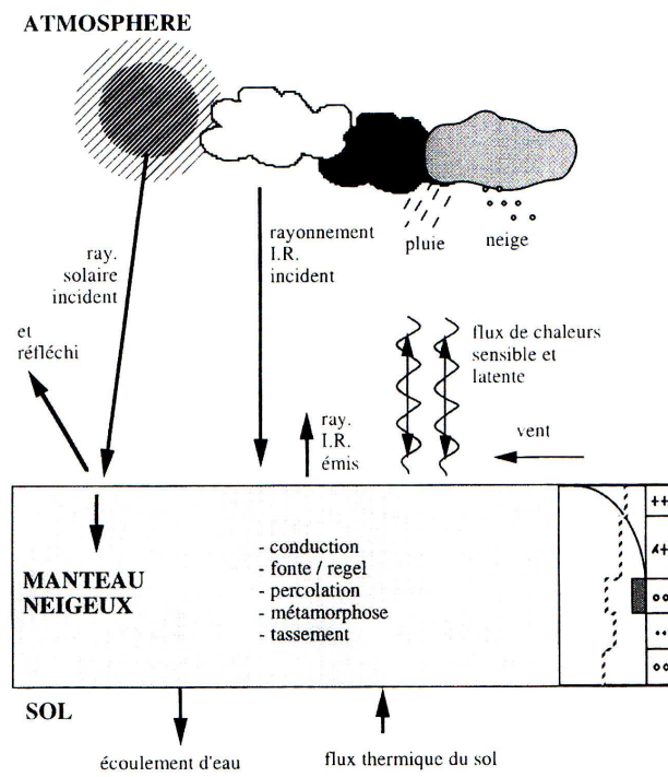
Figure 3.15 Les termes du bilan énergétique du manteau neigeux.
