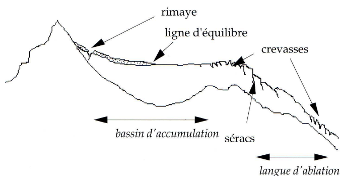
Figure 9.8 Morphologie d'un glacier. C'est l'été que l'on peut le mieux observer et comprendre un glacier car il est le plus souvent à nu, la neige ne persistant qu'en altitude.
