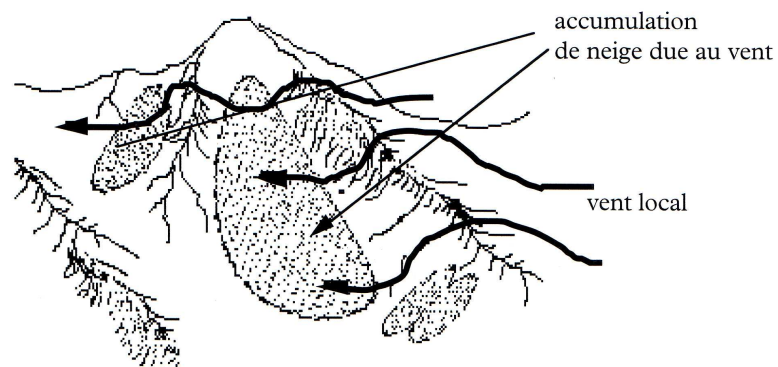
Figure 2.18 La plaque à vent est une accumulation de neige transportée par le vent durant ou après une précipitation.
