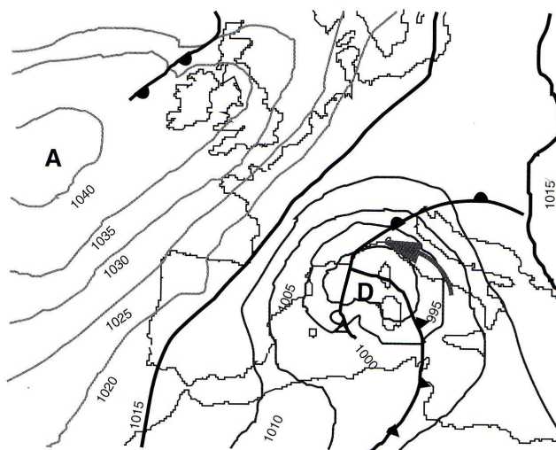
Figure 2.11 Situation dite de retour d'est. Épisode du jeudi 12 janvier 1978 à 18 heures : une dépression située sur la Méditerranée occidentale est en train de se combler, mais un retour d'est (signalé par la flèche) va occasionner d'importantes chutes de neige sur les Alpes (plusieurs avalanches mortelles dans la vallée de Chamonix). D'après [11].
