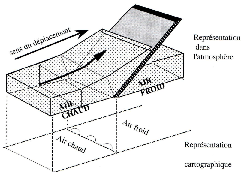
Figure 2.7 Dans le cas d'un front chaud, l'air chaud monte lentement au-dessus de l'air froid. Comme la surface frontale est faiblement inclinée, le front s'étend sur plusieurs centaines de kilomètres. Les cartes météorologiques ne peuvent pas rendre compte de l'étalement de la surface frontale en altitude. Pour le représenter sur une carte, on trace l'intersection de la surface frontale avec le sol. La frontière ainsi délimitée est appelée front chaud, et on la représente comme l'indique la figure, par une ligne continue avec des demi-cercles pointés vers la masse froide. D'après [1].
