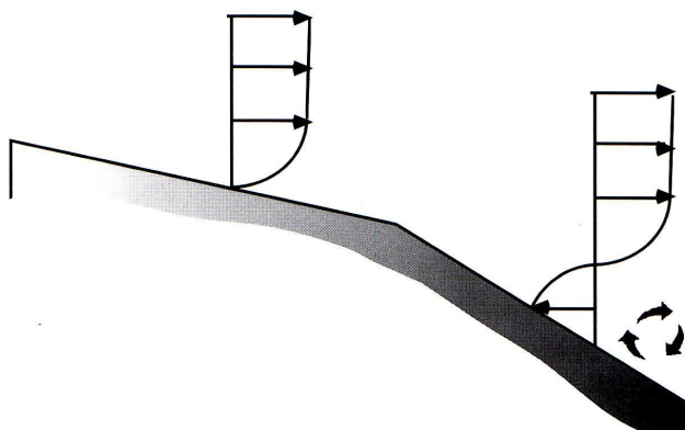
Figure 2.16 Effet d'un changement de déclivité.
