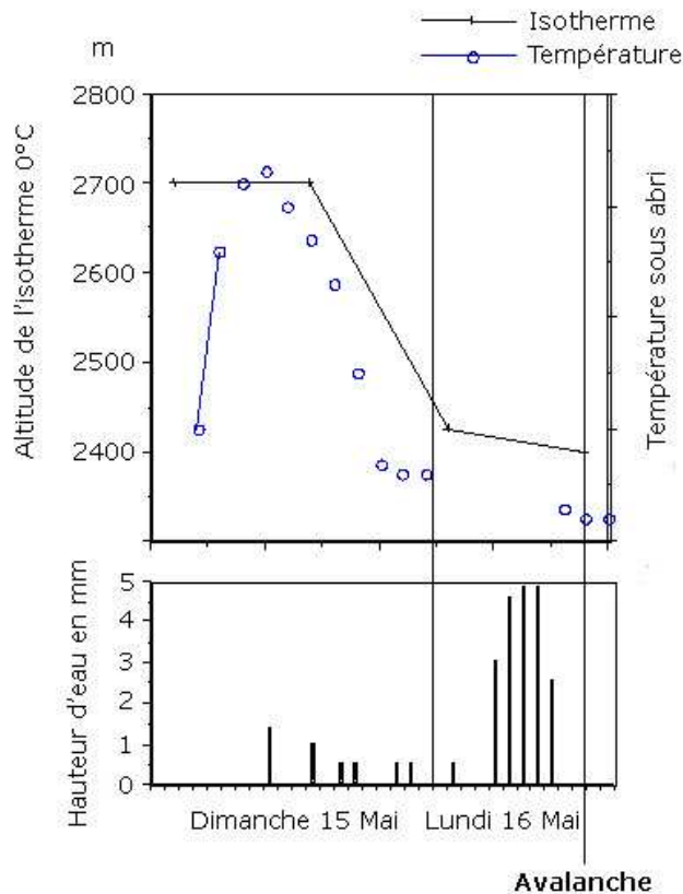
Figure 5.31 Résumé des conditions météorologiques précédant l'avalanche du tunnel du Mont-Blanc (cf. § 5.1.1) : isotherme 0°C (d'après radiosondages de Lyon et Payerne), température (station Nivose des Aiguilles-Rouges, 2330 m), précipitations (recueillies à Chamonix). L'avalanche a eu lieu le 16 mai 1983 à 14h10.
