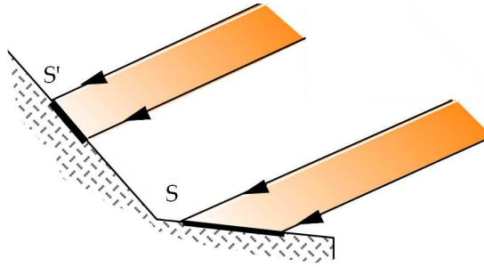
Figure 5.11 Le flux est la quantité de chaleur reçue par unité de surface ; il dépend de l'orientation de la surface par rapport à la direction du rayonnement solaire : le flux est maximal lorsque la surface est perpendiculaire à cette direction.
