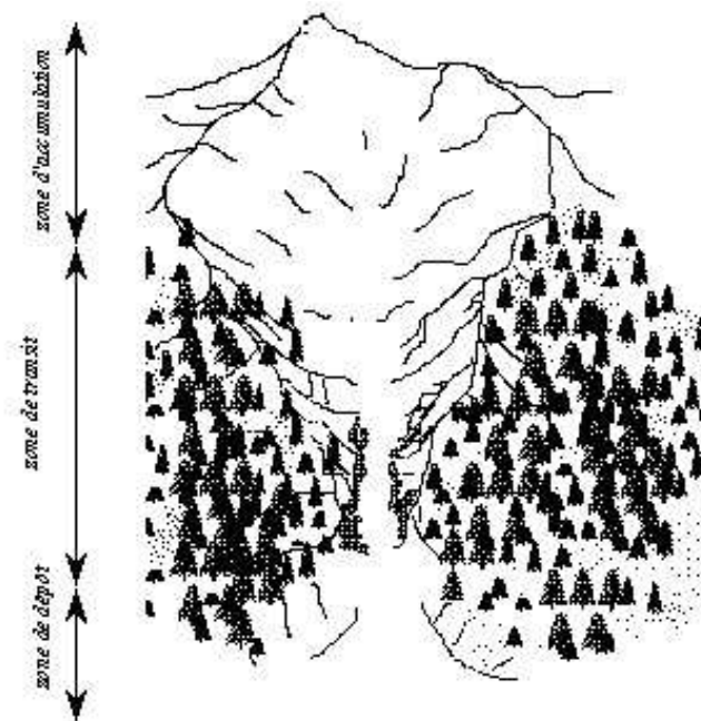
Figure 5.1 Les 3 zones du site. Dans ce cas-ci la troncature est aisée : le cirque constitue la zone d'accumulation, sa forme en entonnoir permet de canaliser l'écoulement dans la zone de transit ; les différentes crêtes découpent des panneaux d'exposition variée. La zone de transit est formée par le ravin d'érosion entre la forêt tandis que la zone de dépôt commence dès que la pente s'affaiblit. Il faudrait préciser également qu'après la description zonale, le spécialiste est amené à introduire des points particuliers tels que des points de rupture de pente, des singularités (ressaut, plateforme, goulot, évasement, obstacle), des lieux remarquables. Mais cela devient une tout autre affaire !
