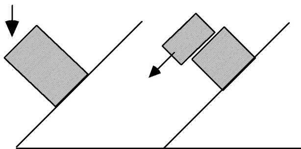
Figure 5.21 Si l'on place une pile de livres sur un plan, il peut rester en équilibre si la pente n'est pas trop forte. Si l'on exerce une force verticale, on amène la pile à la rupture, qui se fera le long de la surface de contact de deux livres.
