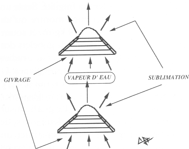
Figure 3.8 Schéma de formation des gobelets.
