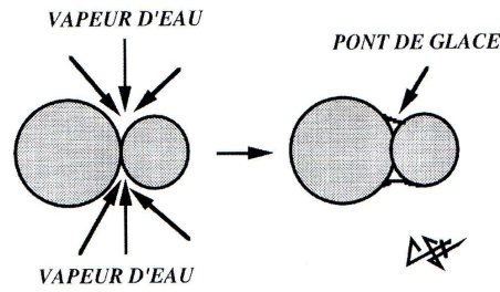
Figure 3.3 Schéma explicatif du phénomène de frittage. La concavité autour du point de contact entre les deux grains est le siège de la condensation solide de la vapeur d'eau.
