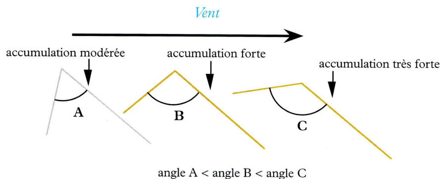
Figure 10.10 Pour des conditions de neige et de vent identiques, l'importance des suraccumulations dépend de la forme du versant « au vent ».
