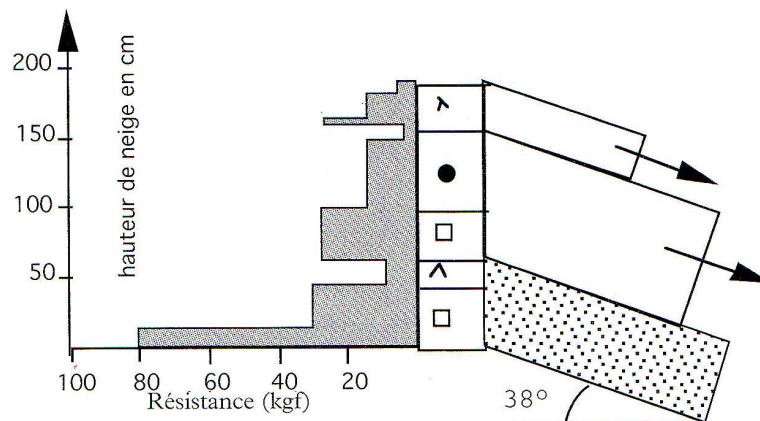
Figure 6.9 Profil simplifié de l'accident de la face nord du Staldenhorn du 6 février 1990 (voir récit chap. 9, § 9.3.2). Le premier décrochement a affecté les 30 premiers centimètres (neige fraîche soufflée); la surface de glissement est constituée par la surface supérieure de l'épaisse couche de grains fins sous-jacente. Le décrochement secondaire a affecté cette couche de grains fins (50 cm d'épaisseur) et une couche de faces planes (environ 40 cm); le glissement s'est effectué à la limite des couches faces planes/gobelets. Un essai de coin suisse indique que la première rupture a lieu après deux sauts (indice de risque e.2 ) et la deuxième après un troisième saut (indice e.3 ). Un test de surface ne permet de détecter que la première instabilité [52].
