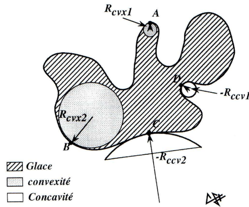
Figure 3.1 Schéma explicatif des rayons de courbure: Le rayon de courbure R_{cvx1} , en A, est le rayon du cercle qui s'inscrit au mieux dans la convexité en A. R_{cvx1} est plus petit que R_{cvx2} et la convexité au voisinage du point A, est plus marquée qu'au voisinage du point B. Pour les concavités aux points C et D, R_{ccv1} est plus petit que R_{ccv2} et la concavité est plus marquée au point D qu'au point C.
