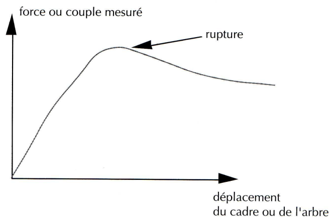
Figure 6.5 La détermination de la résistance au cisaillement se fait en mesurant la force (ou le couple) à la rupture. Généralement, la rupture se traduit dans un diagramme force-déplacement (ou couple-rotation) du cadre par l'existence d'un maximum. Le passage de la valeur de la force maximale à la valeur de la résistance fait généralement appel à des facteurs de correction, qui varient selon les auteurs.
