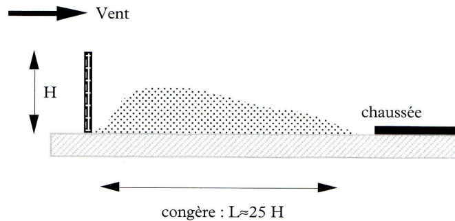
Figure 8.5 Effet dû à un obstacle poreux sans garde au sol. D'après [8].
