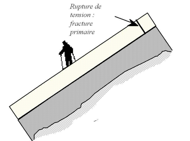
Figure 5.33 Le passage d'un skieur (composante tangentielle du poids) provoque une augmentation des tensions au sein de la couche superficielle, qui se tend (un peu à la manière d'un ressort). Pour contrebalancer la force imposée, la tension doit se propager sur de grandes distances.
