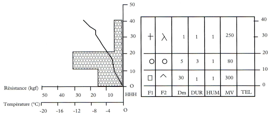
Figure 4.2 Type de représentation préconisé par Météo-France. HHH désigne la hauteur de neige en cm, F1/F2 le type de grains majoritaires/minoritaires, Dm le diamètre moyen, DUR et HUM les indices de dureté et d'humidité, MV et TEL, les mesures de masse volumique et de TEL.
